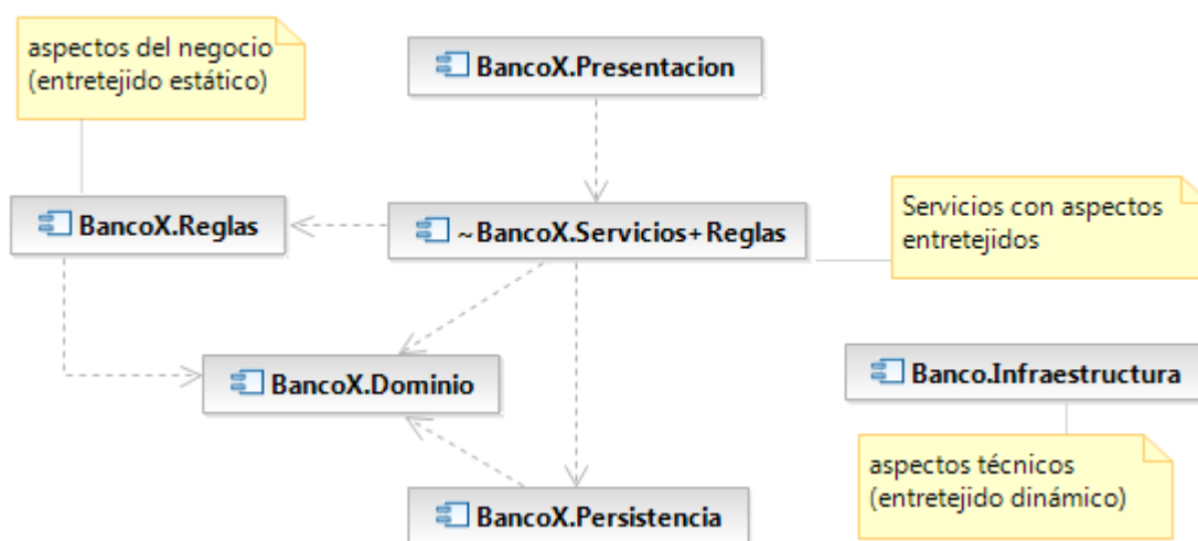
Figura 67: ssemblies de la solución AOP luego del entrelazado
