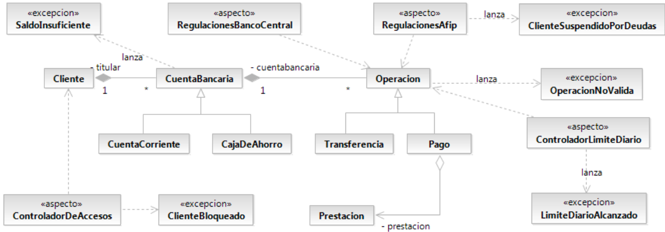
Figura 64: clases del domino extendidas con aspectos del negocio del Banco X
