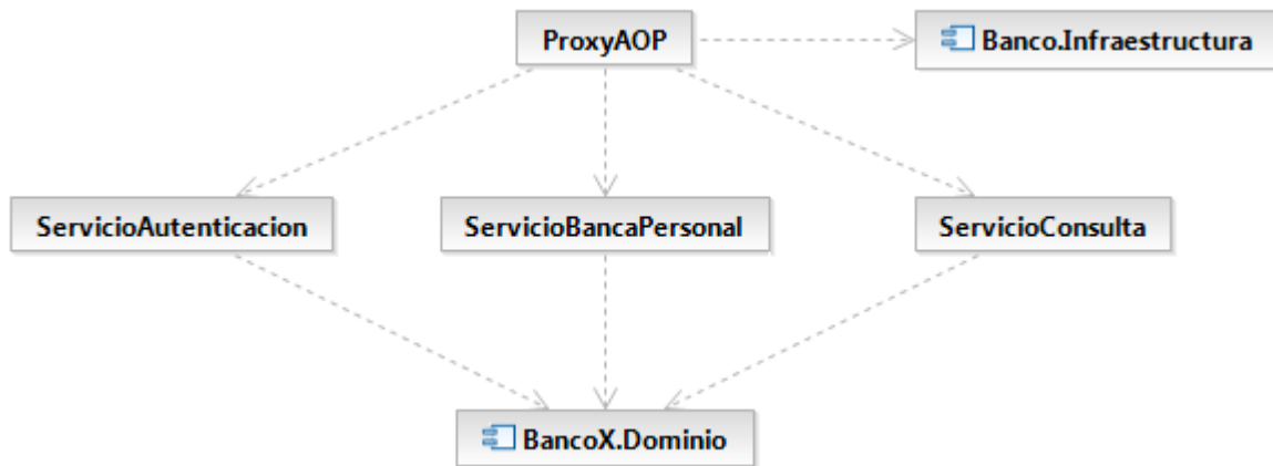
Figura 65: Clases de la capa de servicios con aspectos de infraestructura
